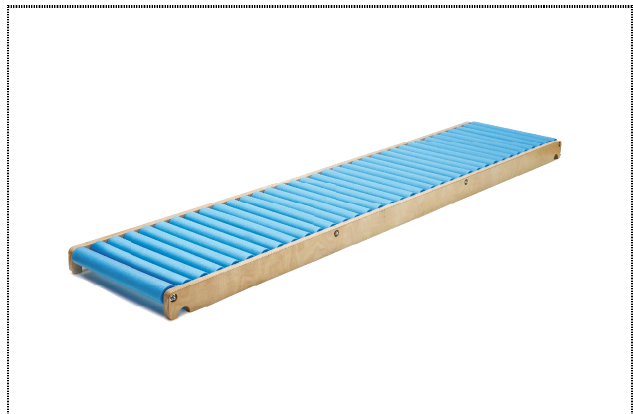
Abbildung 4: Rollenrutsche L Art.-Nr. 44441, Abmessungen <bodenliegend> ca. 251,0 x 57,5 x 9,4 cm (L x B x H)
