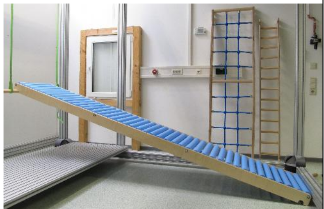
Abbildung 2: Rollenrutsche XL Art.-Nr. 44444 (7016-15-G/012), Abmessungen ohne Schaumstoffrollen <bodenliegend> ca. 299,0 x 56,5 x 9,5 cm (L x B x H)
