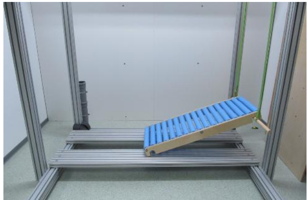
Abbildung 8: Rollenrutsche S Art.-Nr. 44465 (7003-12-G/004), Abmessungen <bodenliegend> ca. 116,5 x 57,5 x 9,4 cm (L x B x H)
