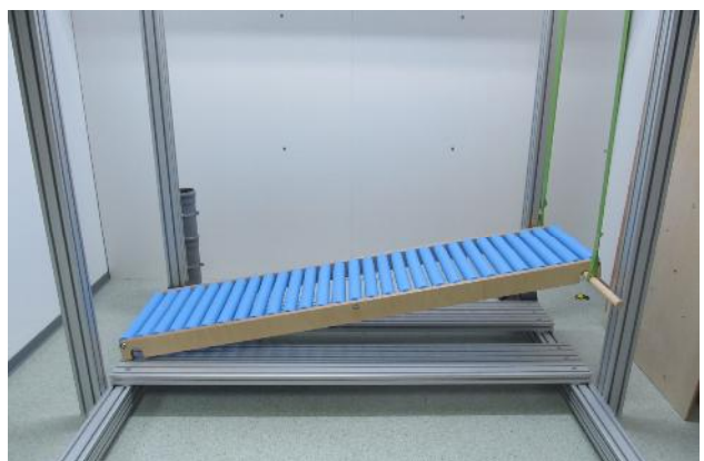
Abbildung 6: Rollenrutsche Art.-Nr. 44464 (7003-12-G/003), Abmessungen <bodenliegend> ca. 205,5 x 57,5 x 9,4 cm (L x B x H)
